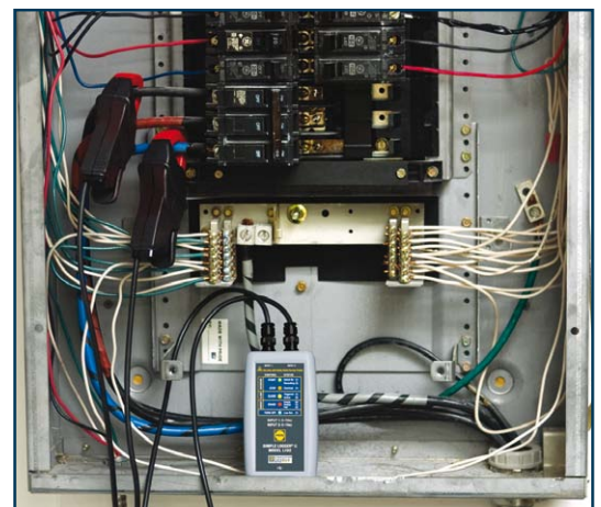
Stromaufnahme an 2 Außenleitern mit L102.
